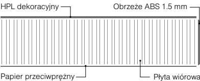
Obrzeże ABS
